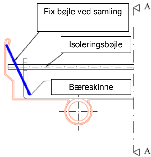
Sektion A-A
